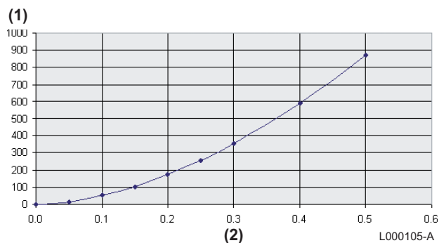
(1) Tlaková ztráta (mbar) (2) Objemový průtok (m³/h)
