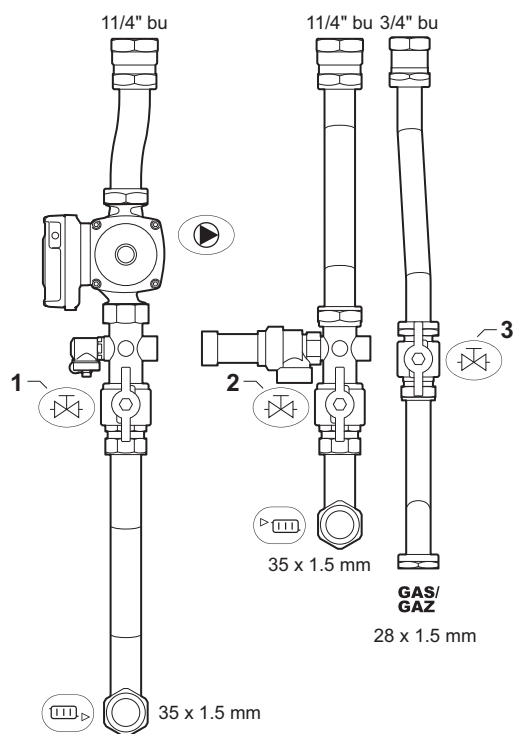
Obr.6 Připojovací sada s čerpadlem MCA 45-115
