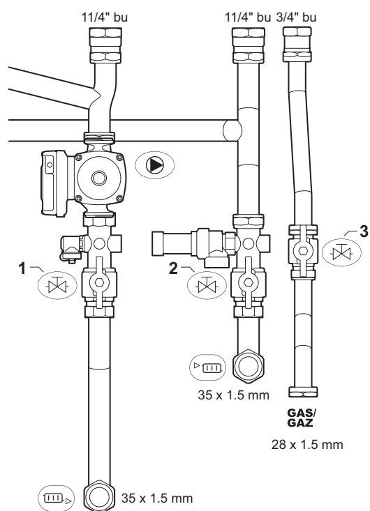
Obr.8 Připojovací sada pro ohřívač MCA 45-115
