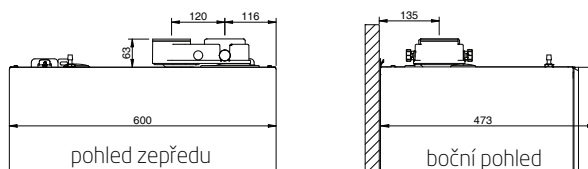
Vivadens MCR...BIC
