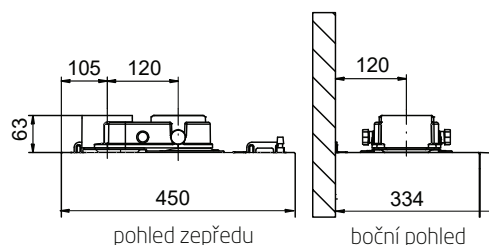
Virtuens MCA
